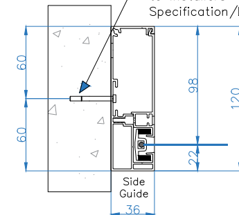
Side Fix Guide
