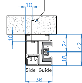
Face Fix Guide
